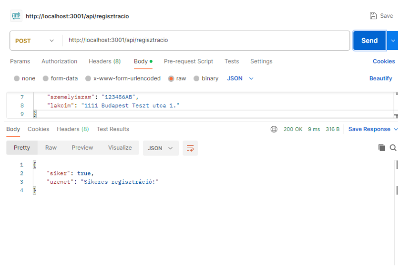
1.Részlet a regisztracio.js fájl Postman teszteléséből.
