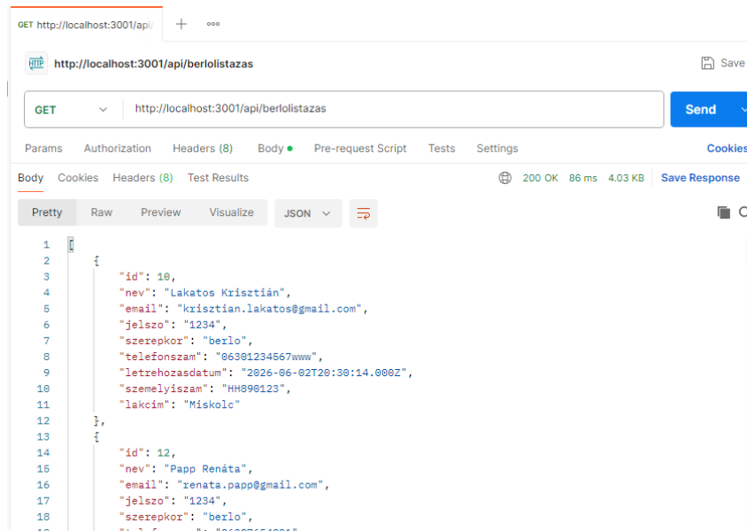
1.Kép: Bérlok listázásának Postman tesztelése.
