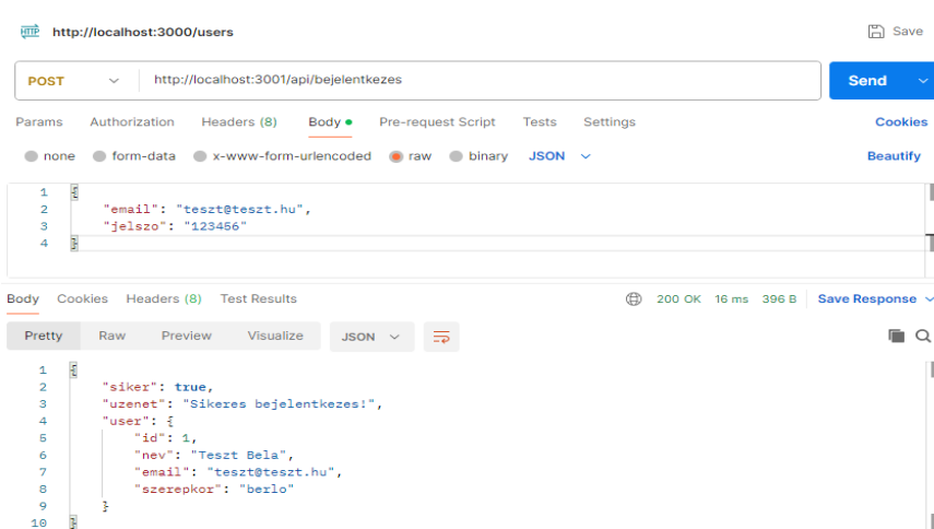
2. Részlet a bejelentkezés.js fájl Postman teszteléséből.
